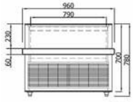
309114 Seitenskizze
